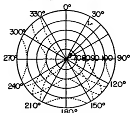
(g) 50 mi. PPI, delayed 60 mi.; 20 mi. grid. Note extreme distortion.
