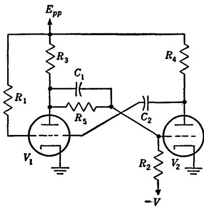
FIG. 4-23.—Flip-flop circuit.
