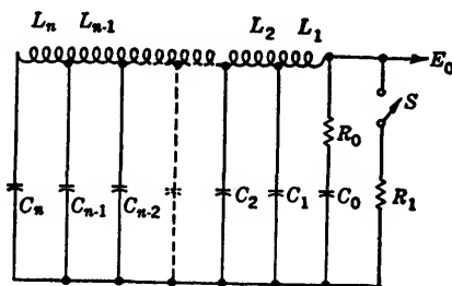
Fig. 7-25.—Intensifier circuit.
