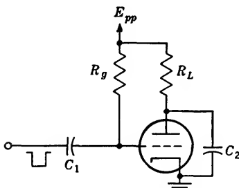
FIG. 4-1.—Triode amplifier.
