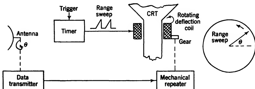
Fig. 1-9.—Rotating-coil PPI.
